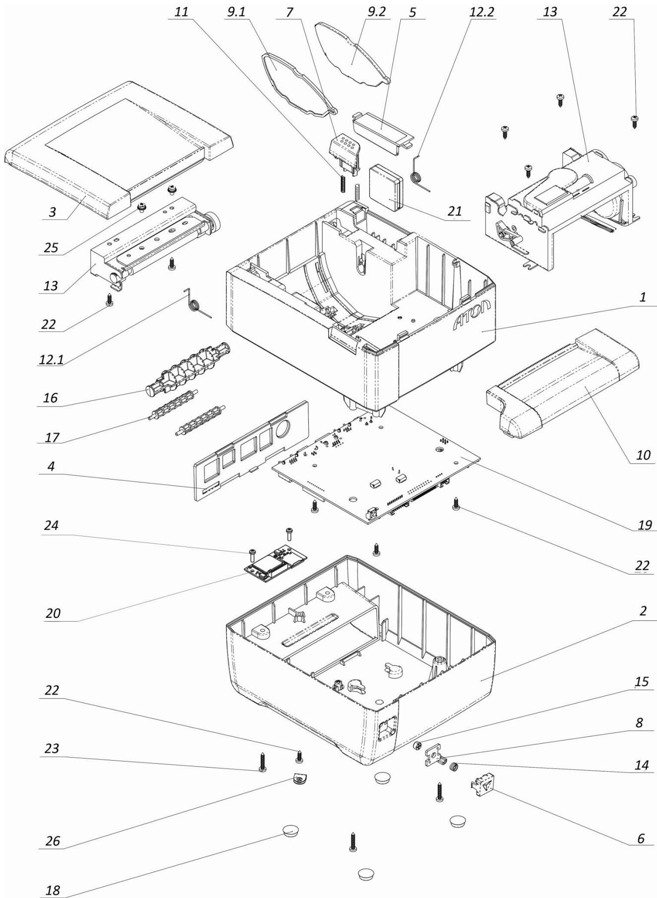
Рисунок 1. Компонировочная схема ККТ АТОЛ 25Ф
